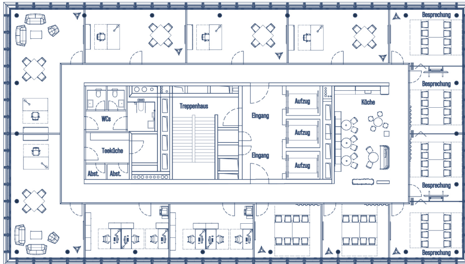
ENTWURFSPLANUNG MANAGEMENTETAGE
