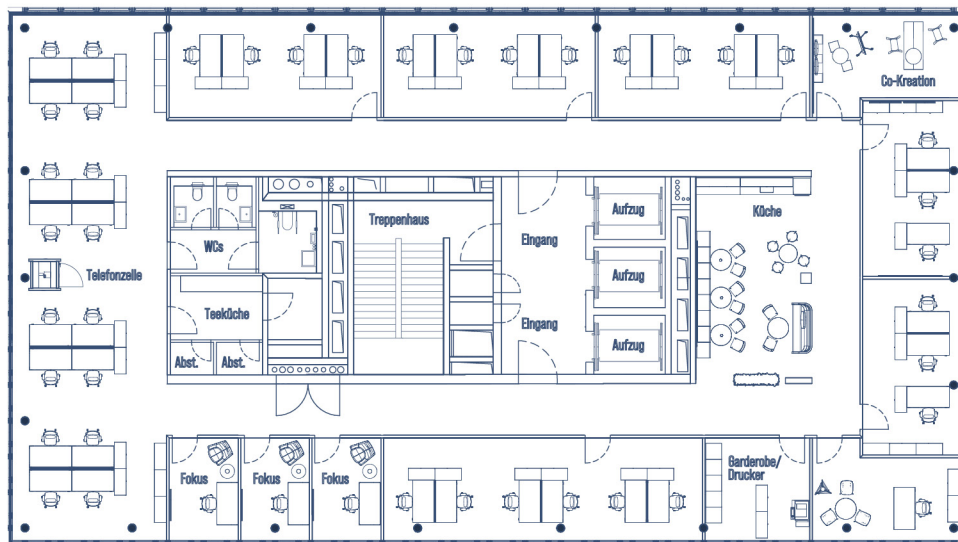
ENTWURFSPLANUNG BÜROETAGE CLASSIC
